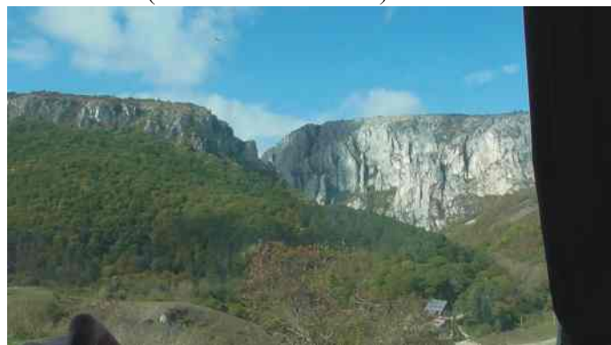
Tordai-hasadék
